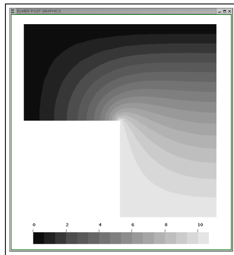
Kuva 4: Lämpötilajakauma
